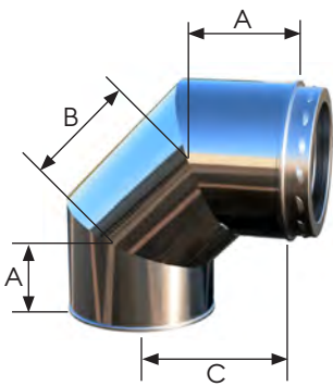
85°, 87° & 90° Elbows
