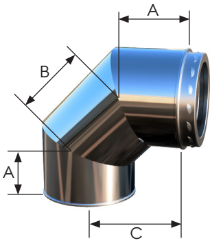
85°, 87° & 90° Elbows
